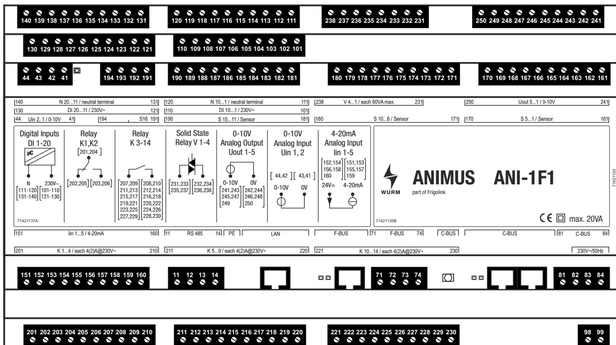
Abb. 2: ANI-1F1 - Schaltbild
