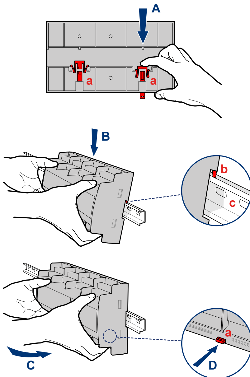
Abb. 6: ANI-1F1 - HutschieneMontage
