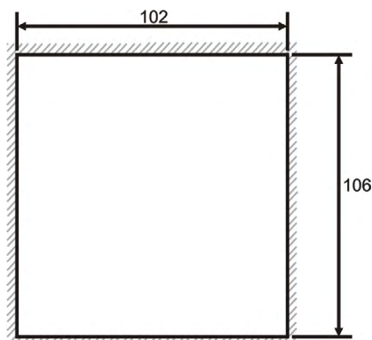
Einbauausschnitt für Einzelmontage
