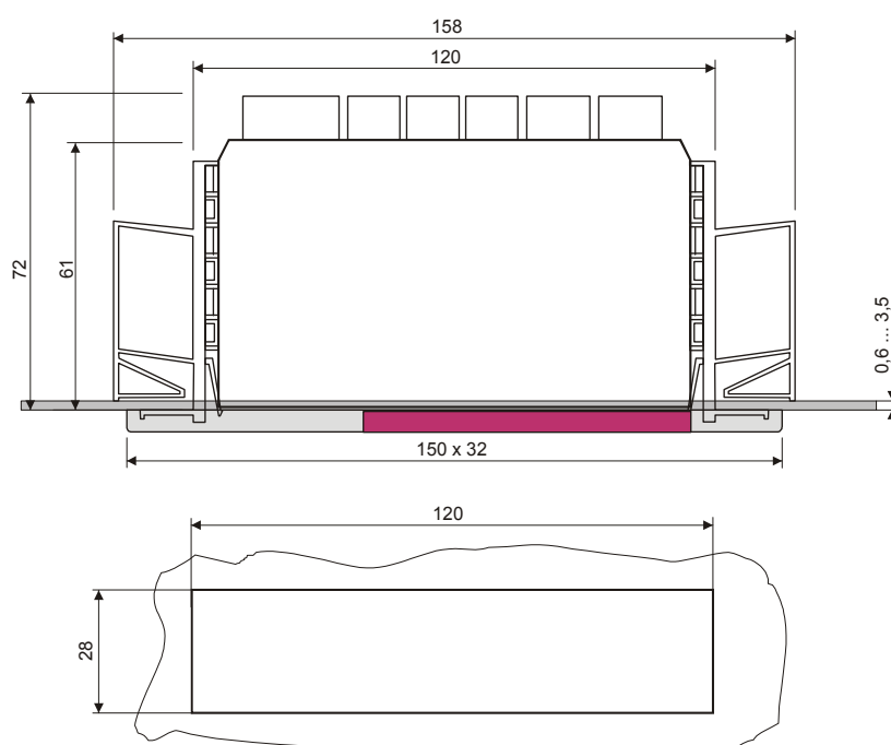
Einbauausschnitt
