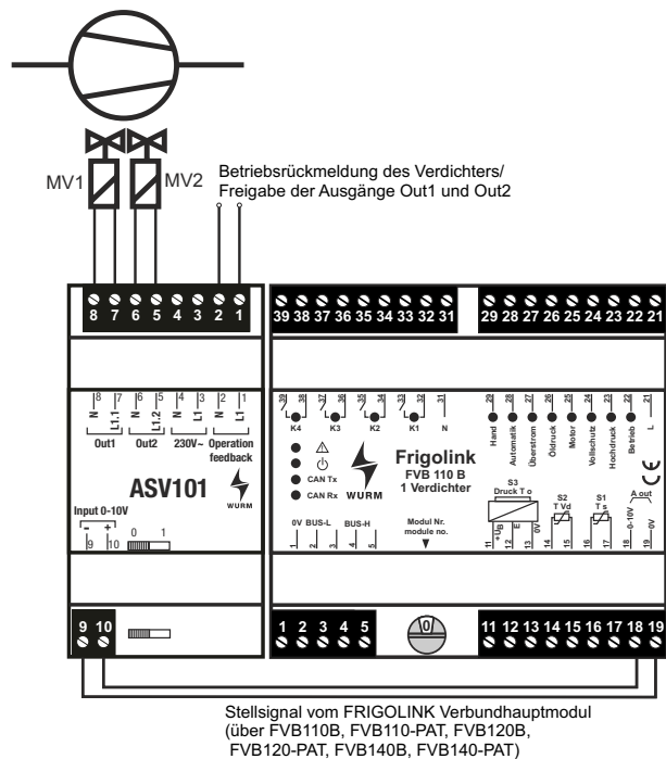
Abb. 2: ASV101 - Schaltbild
