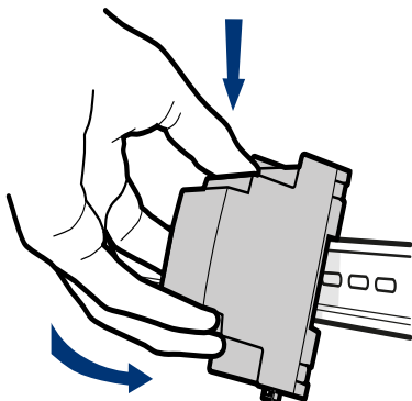
Abb. 4: ASV101 - Hutschienenmontage
