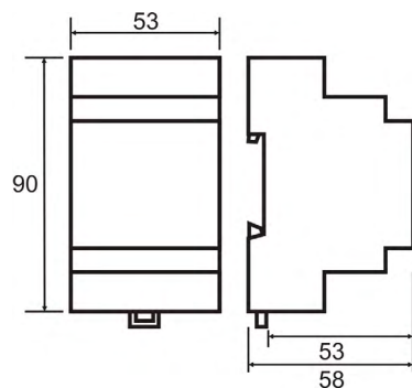
Abb. 3: ASV101 - Abmessungen
