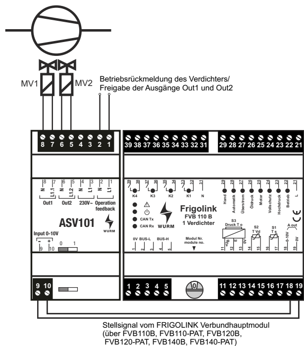
Abb. 2: ASV101 - Schaltbild
