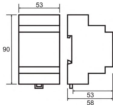
Abb. 3: ASV101 - Abmessungen
