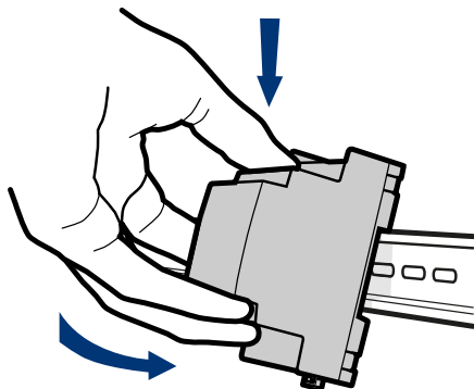
Abb. 4: ASV101 - Hutschienenmontage
