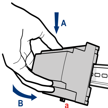
Abb. 3: Hutschiennenmontage
