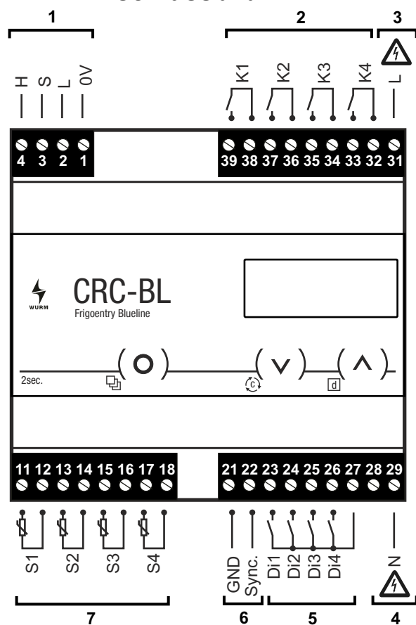
Abb. 2: Anschlussbild
