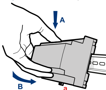
Abb. 3: Hutschiennenmontage
