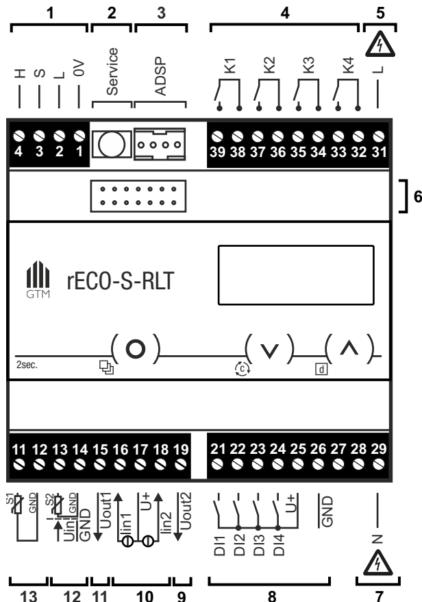
Abb. 2: Anschlussbild
