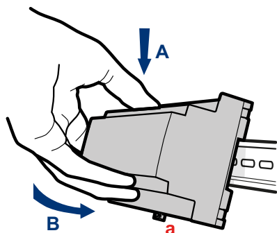
Abb. 3: Hutschiennenmontage
