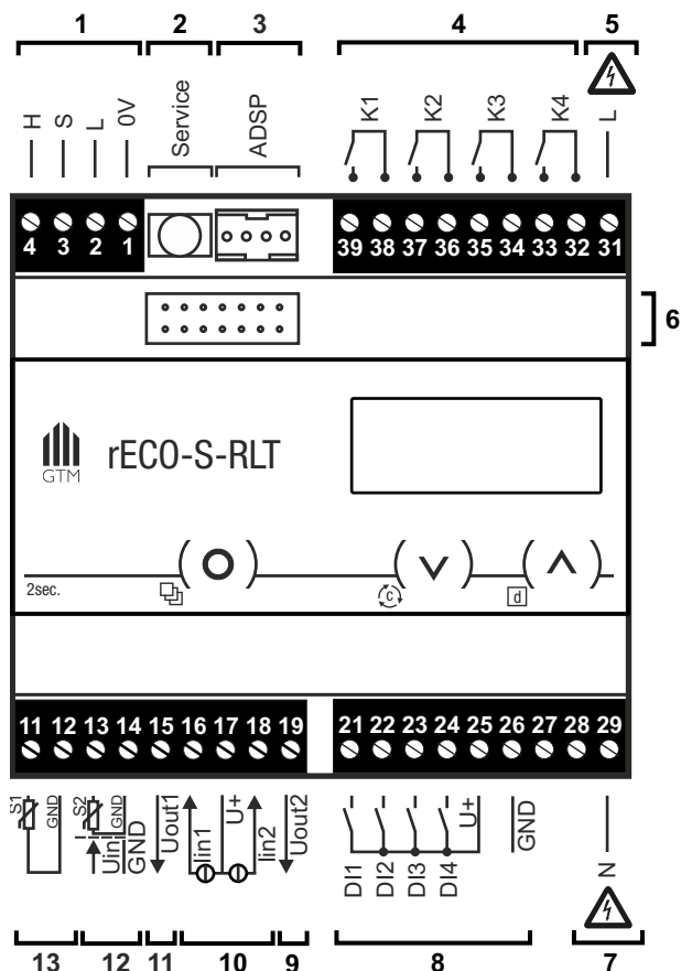
Abb. 2: Anschlussbild
