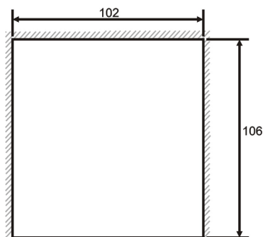
Einbauausschnitt für Einzelmontage
