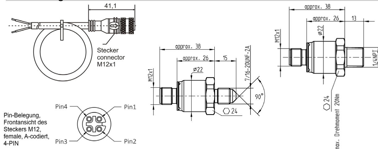
Abb. 3: DAR 7...DAR 120
