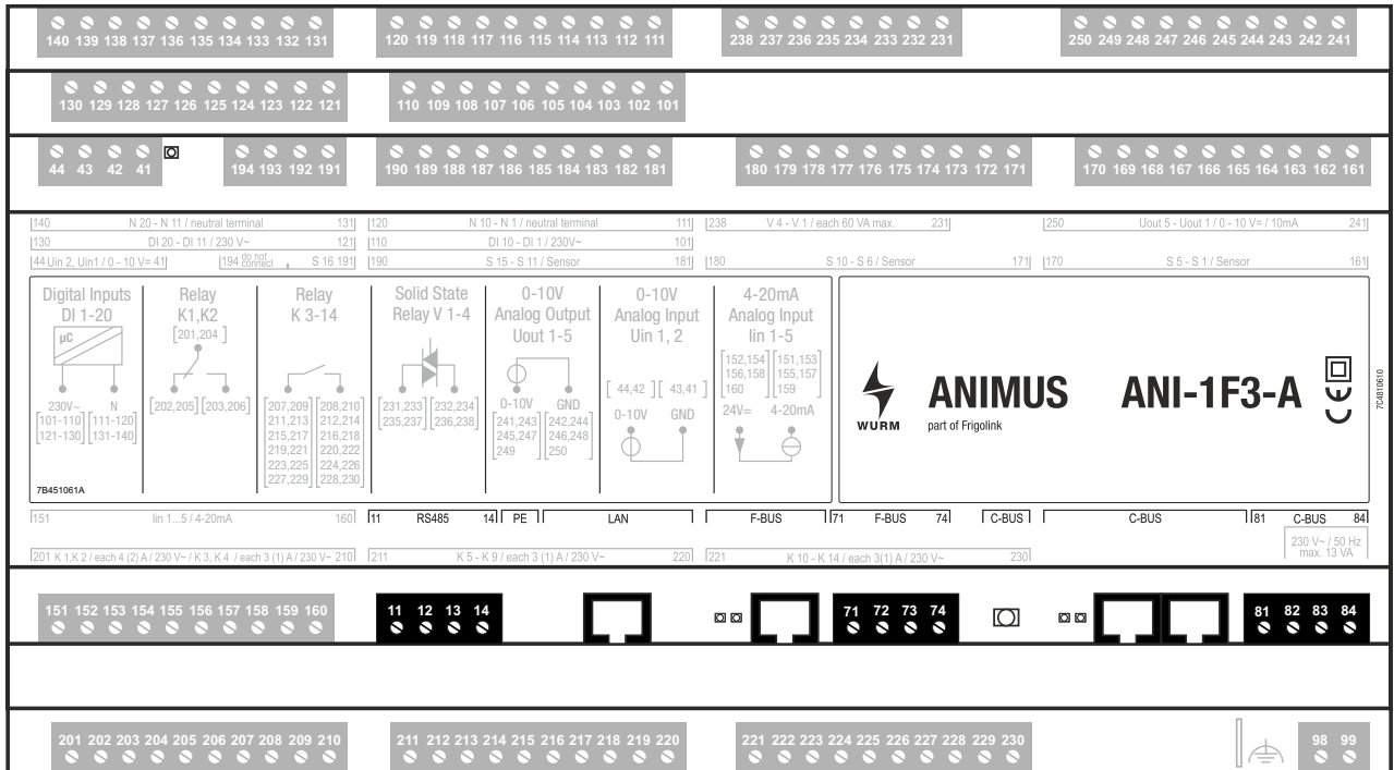
Abb. 5: Schaltbild Kommunikation
