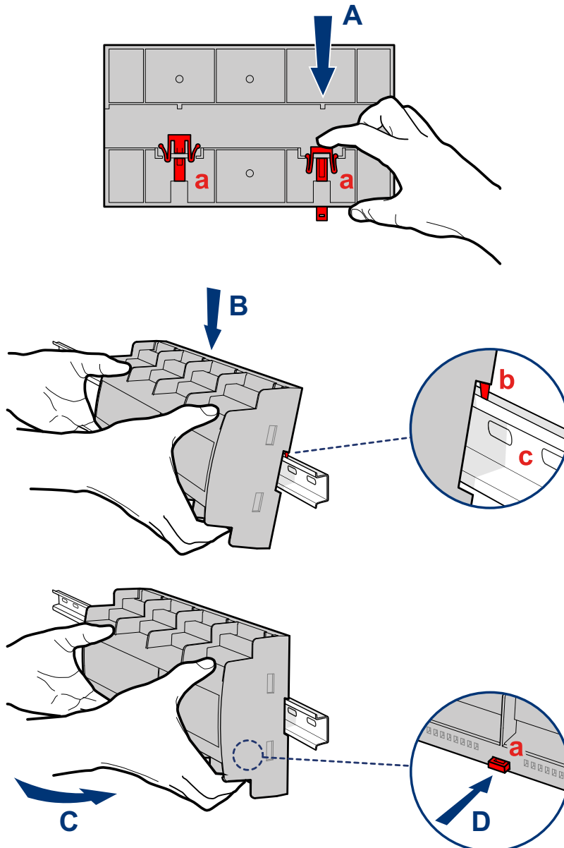
Abb. 8: HutschieneMontage
