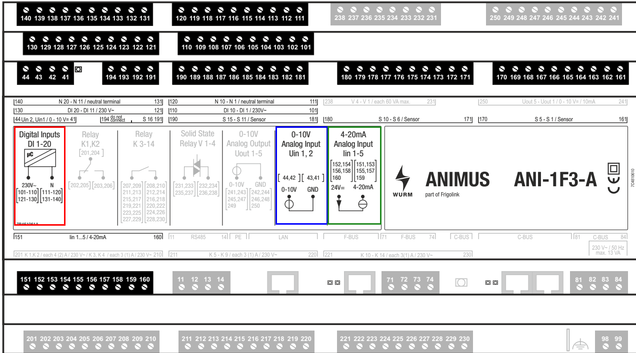
Abb. 3: Schaltbild Eingänge
