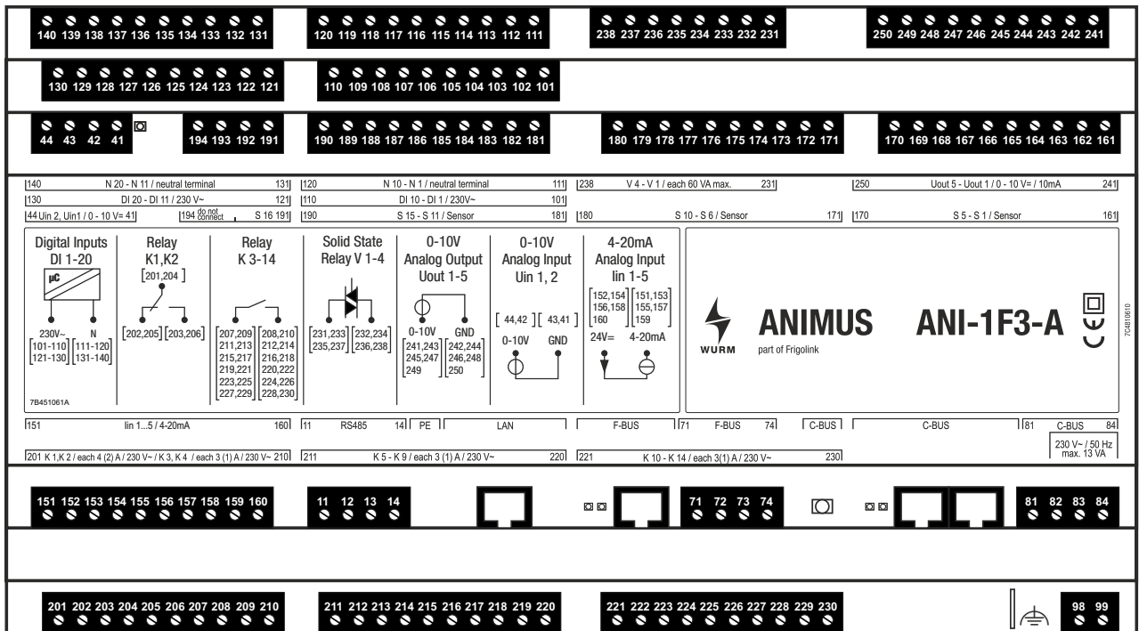
Abb. 2: Schaltbild
