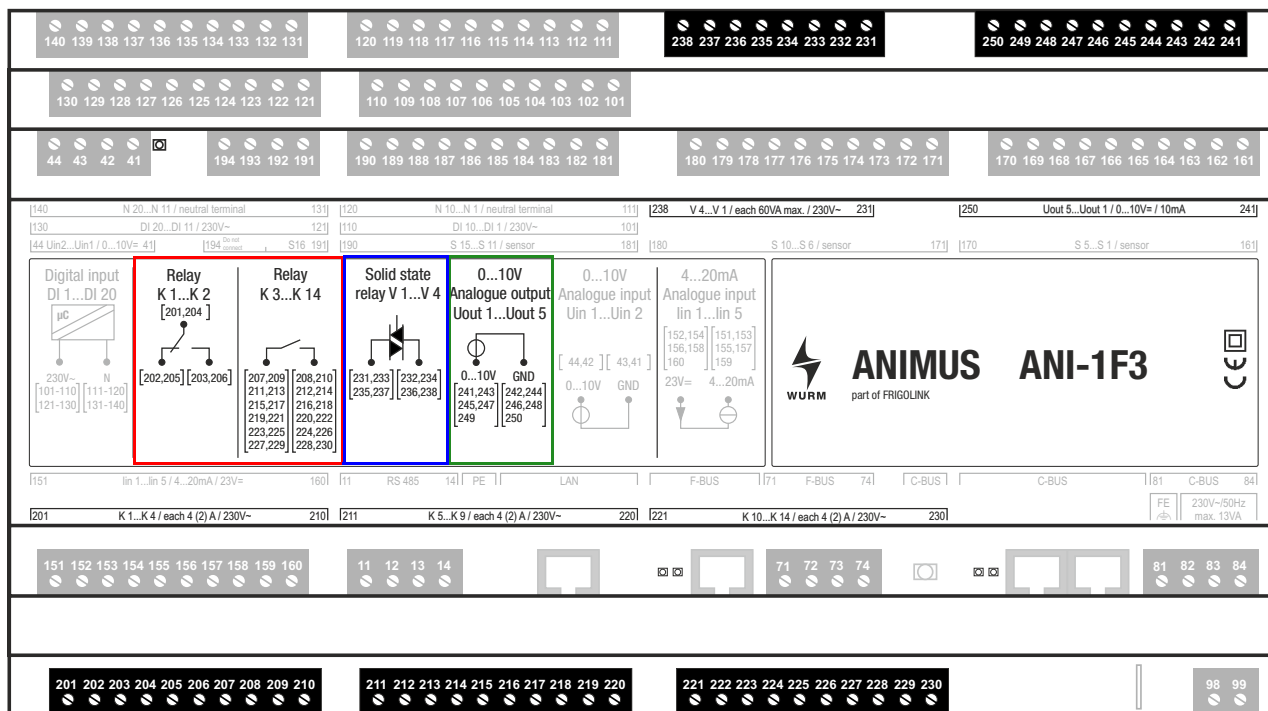
Abb. 4: ANI-1F3 Schaltbild Ausgänge
