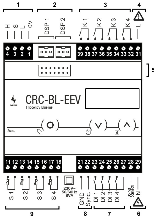
Abb. 2: Anschlussbild
