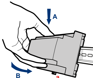
Abb. 3: Hutschiennenmontage
