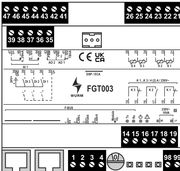
Abb. 2: Anschlussbild
