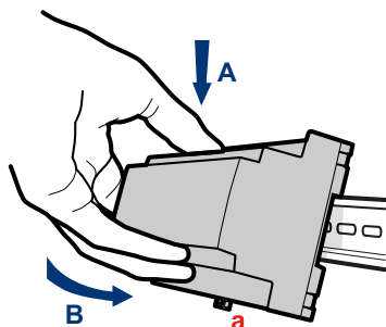
Abb. 3: Hutschienenmontage
