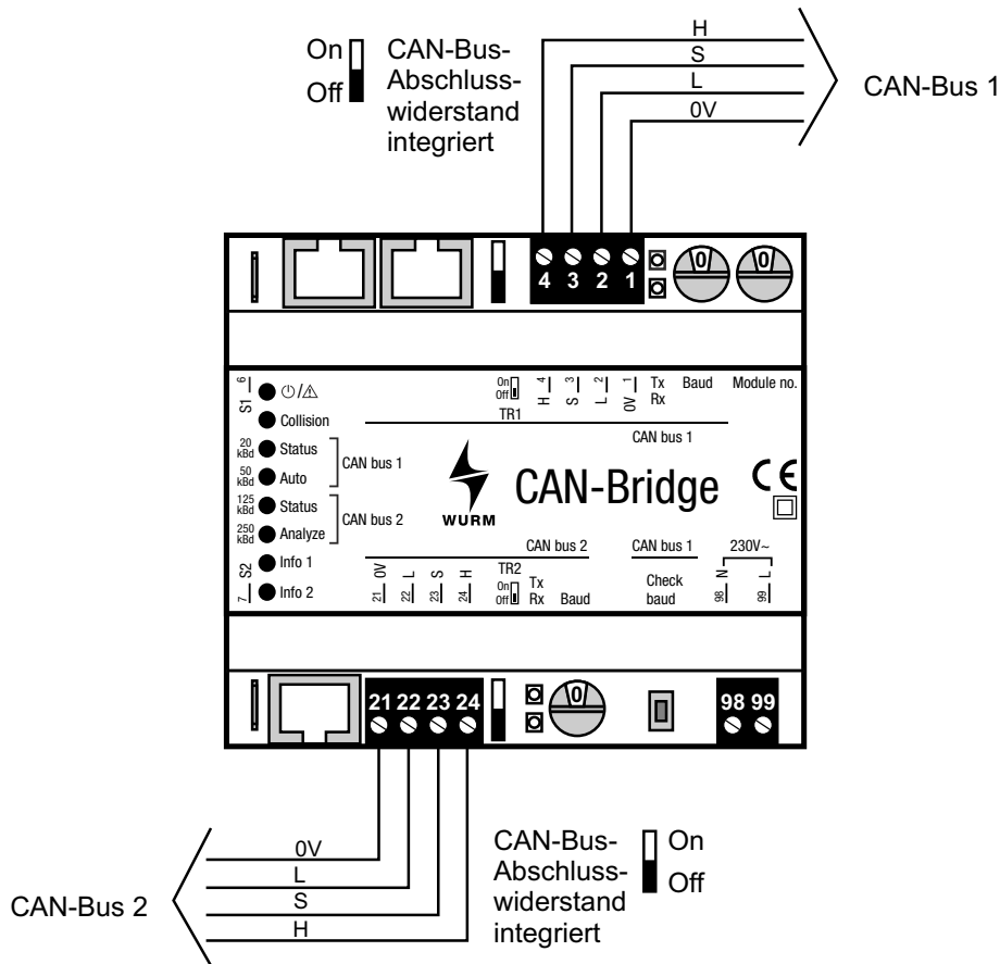
Abb. 3: Anschlussbild
