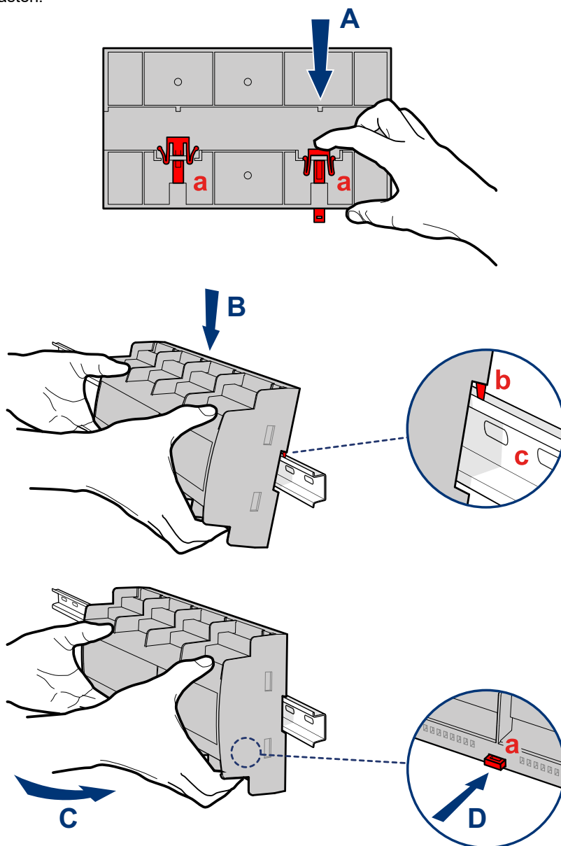
Abb. 8: ANI-1F3 - Hutschienenmontage
