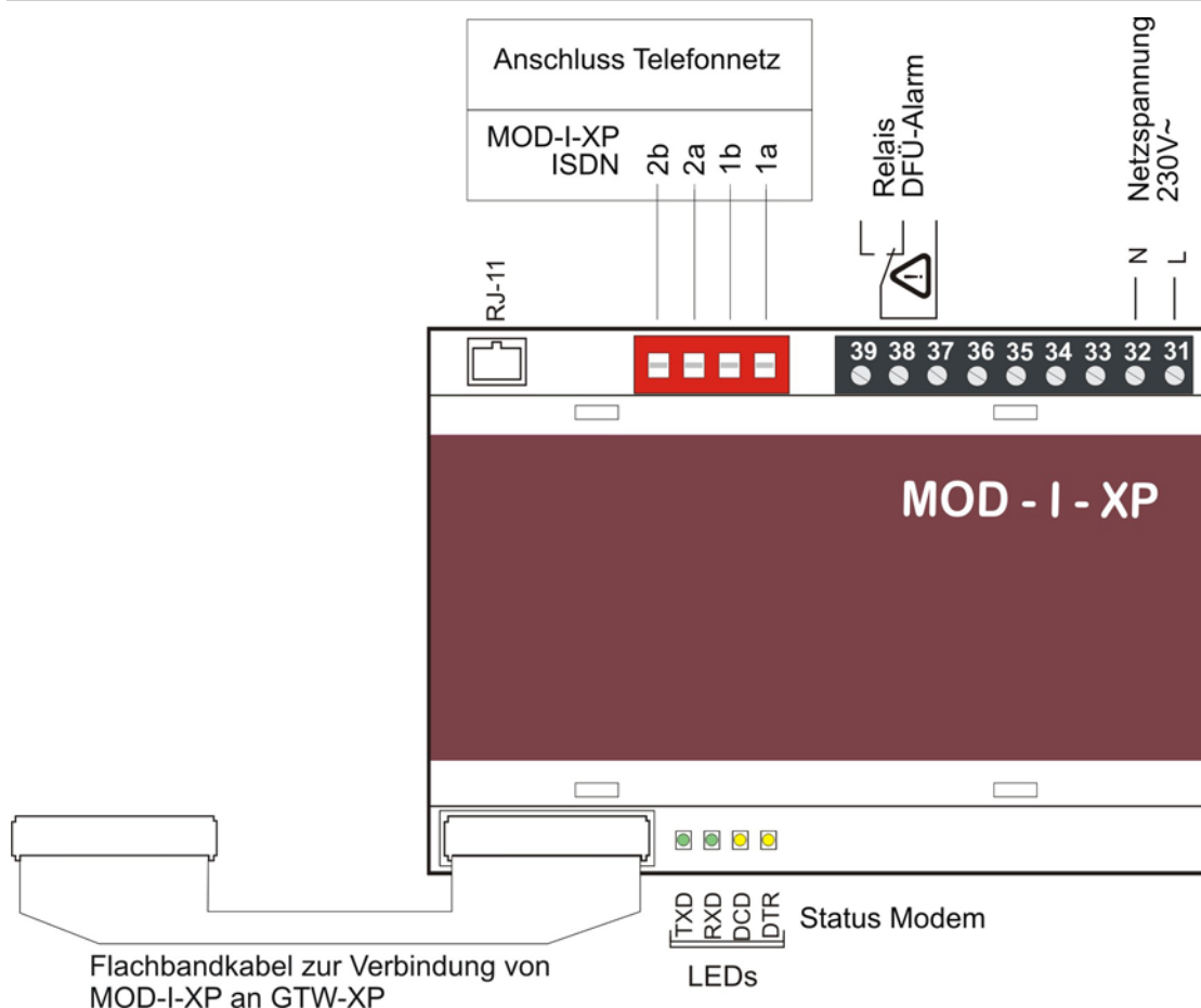
Abb. 1 Schaltbild MOD-I-XP
