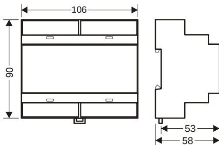
Abb. 2 Abmessungen MOD-I-XP
