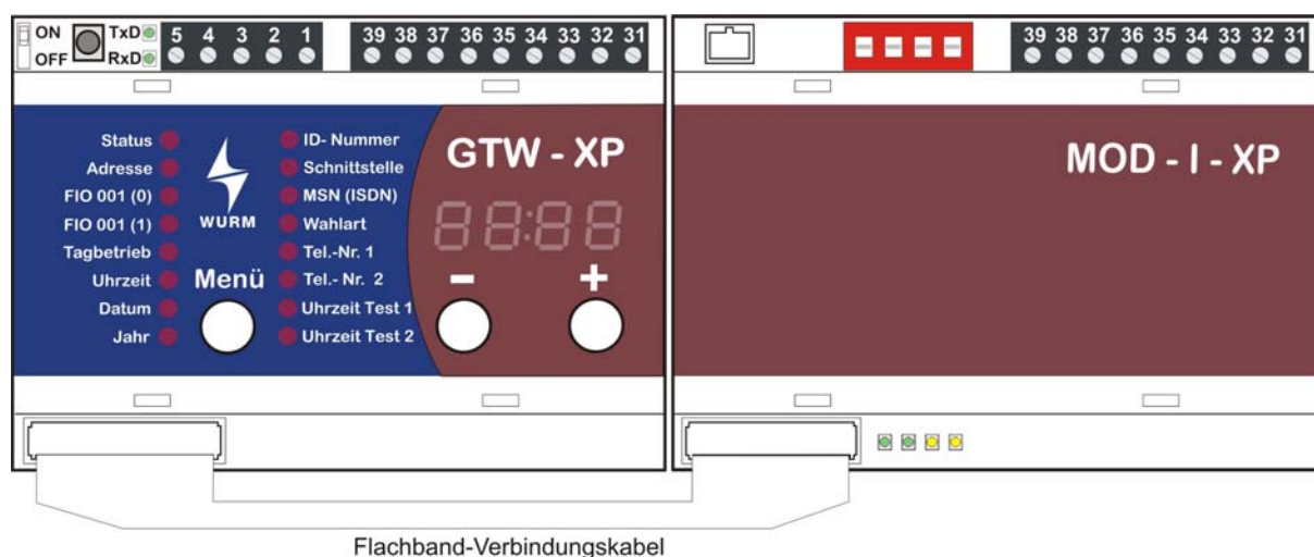
Abb. 4 Anschlussbild GTW-XP an MOD-I-XP
